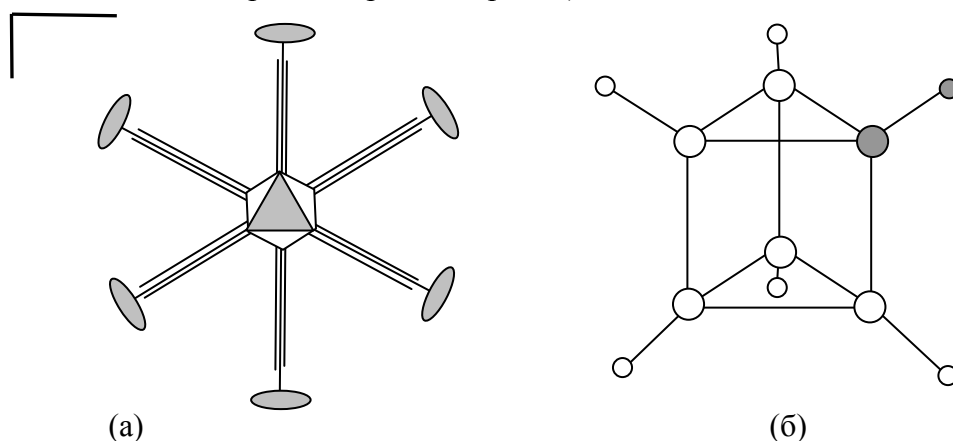
Рис. 1.11. (а) График группы \bar{6}m2 (нанести орбиты). (б) Молекула призмы («дьюаровского бензола») C_6H_6 ( \bar{6}m2 ): выделена симметрически независимая часть.
