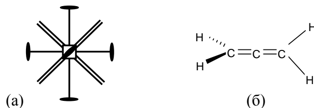
Рис. 1.8. (а) График группы \overline{4}2m ( D_{2d} ), (б) молекула аллена, обладающая этой симметрией
